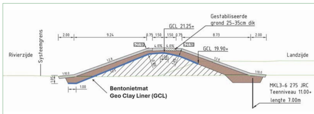
Figuur 11 – Typerend dwarsprofiel dijkversterking Beesel, met positie van de bentonietmat in gestreepte blauwe lijn op het buitendijks talud, kruin en gedeelte binnendijks.
