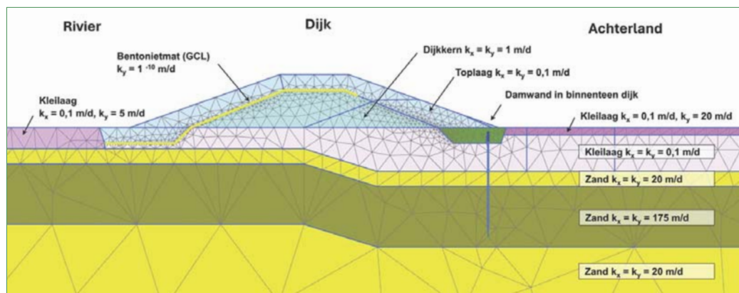
Figuur 10 – Overzicht van schematisatie van de dijk in PLAXIS met bentonietmatten in de stromingsberekningen die zijn uitgevoerd om de geohydrologische situatie bij maatgevende omstandigheden te bepalen, inclusief de gebruikte doorlatendheidsfactoren (k-waarde in m/dag).
