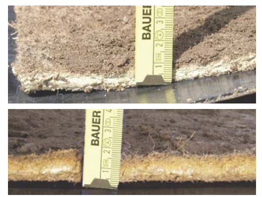
Figuur 16a en b – Detail monsternamen gehydrateerde bentonietmat bij de Elbe dijk Wittenberge met analyse van mechanisch en fysische veranderingen vanuit BAW Duitsland.
